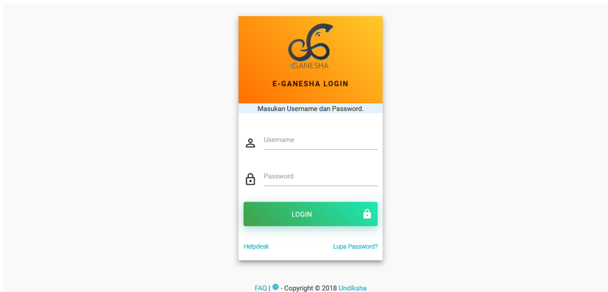
Gambar 2. Login SSO
