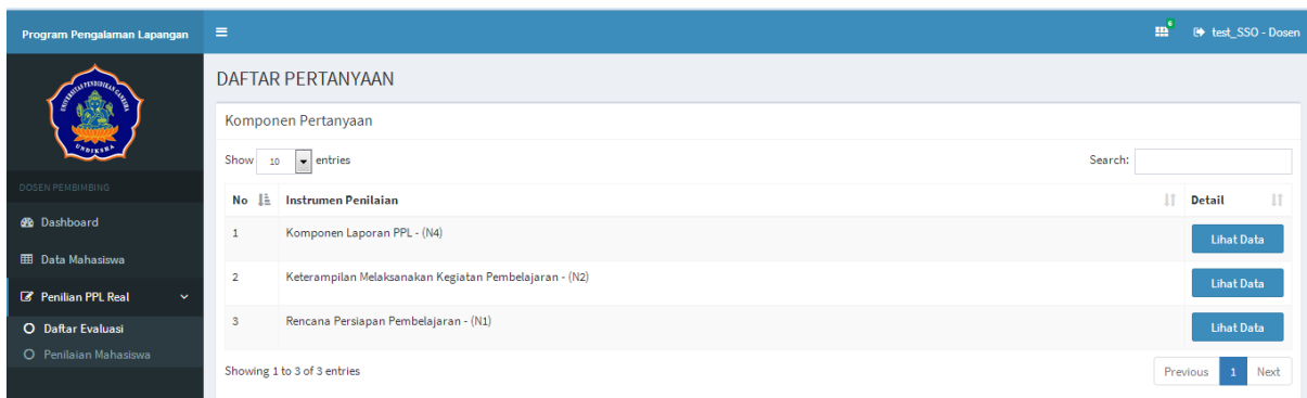
Gambar 25. Daftar Evaluasi
