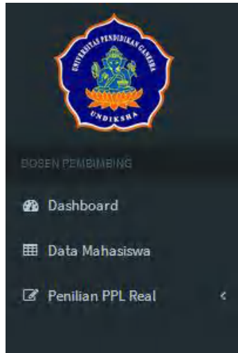
Gambar 24. Menu Pembimbing
