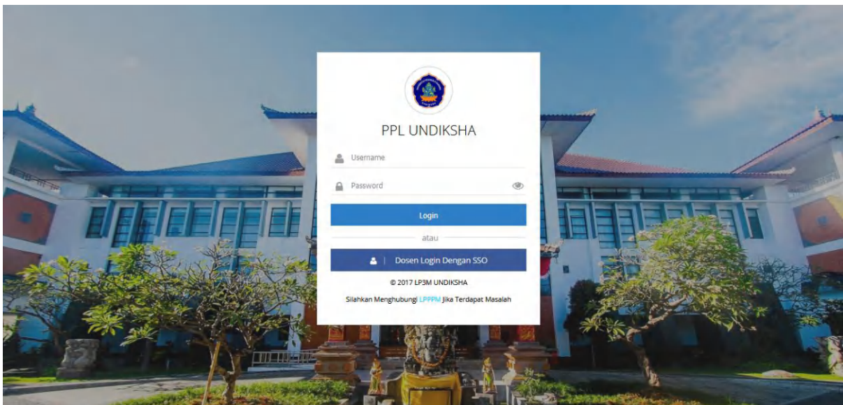
Gambar 1. Halaman Login
